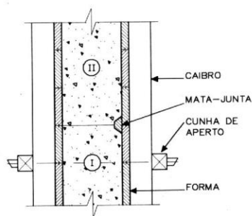
DESENHO 3
